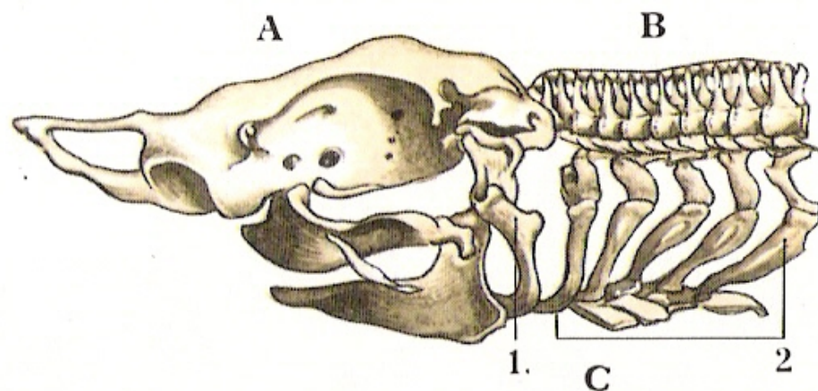
Obr. 154. Schéma žraločí lebky A mozková schránka s čichovou, zrakovou a sluchovou oblastí, B páteř, C kostra útrobní, 1 oblouk patročelistní a jazylkový, 2 oblouky žaberní
